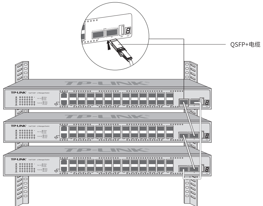
图2-4 使用QSFP+端口建立堆叠示意图
