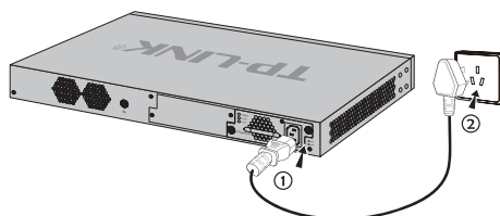
图3-4 电源线连接示意图
