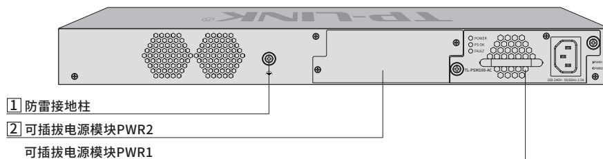
图1-2 TL-ST7226F后面板示意图
