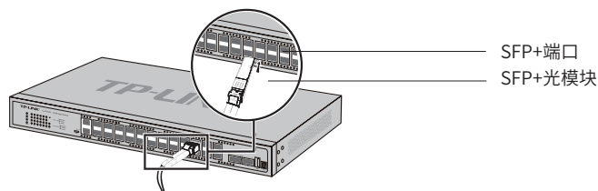
图3-1 SFP+端口连接示意图
