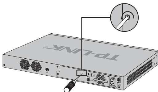
图3-5 移除保护面板示意图
