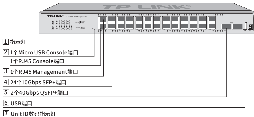
图1-1 TL-ST7226F前面板示意图
