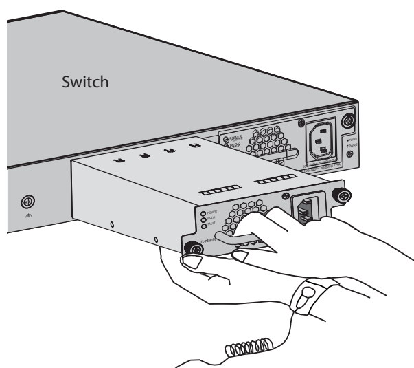
图3-6 安装电源模块示意图
